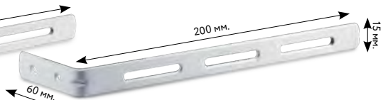
АДАПТЕР ДЛЯ ЭКРЕРНОГО УГЛА 3-Х РЯДНЫЙ
