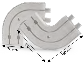
ЭКРЕРНЫЙ УГОЛ 3-РЯДНЫЙ ВНЕШНИЙ
