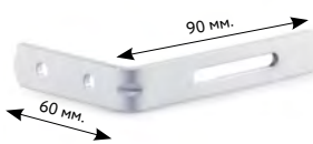
ПЛАСТИНА ДЛЯ КРОНШТЕЙНА СТЕНОВОГО
