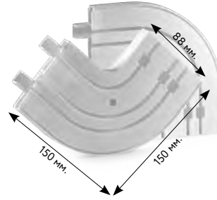
ЭКРЕРНЫЙ УГОЛ 2-РЯДНЫЙ ВНУТРЕННИЙ
